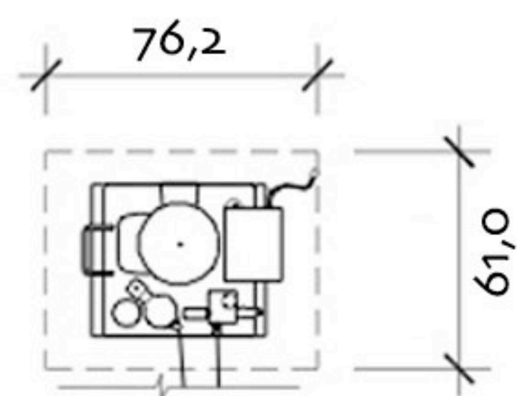
Unità idraulica (dimensioni di ingombro)
