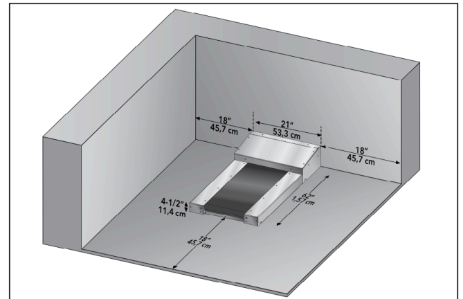
Misure tapis roulant
